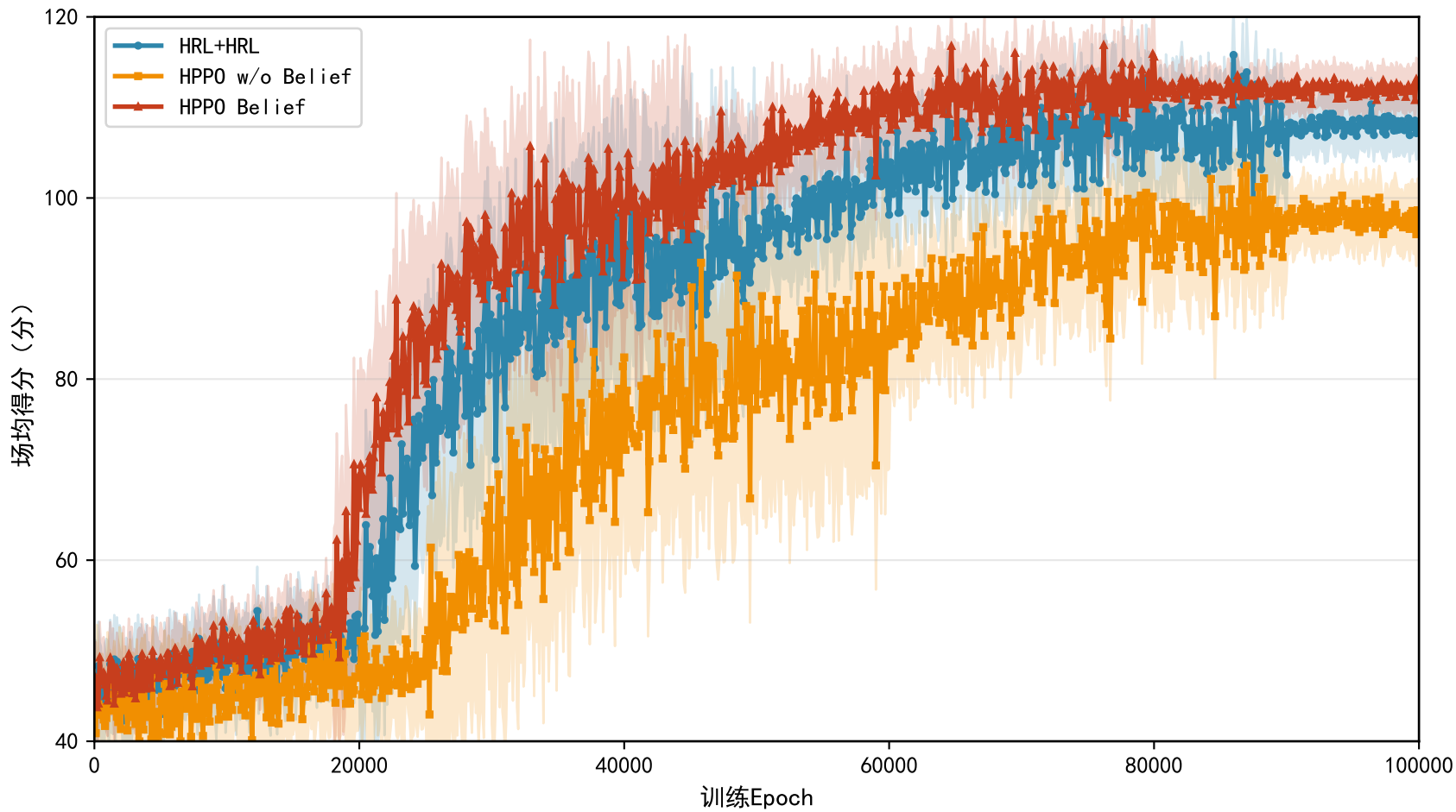
多模型训练得分收敛曲线对比（对战RuleRobot+RuleRobot）
